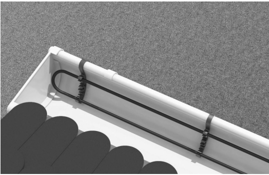
Крепеж для желобов GH-2
