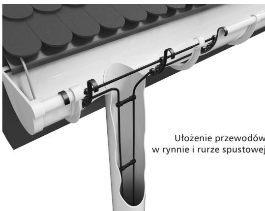
Linka z uchwytami do rur spustowych DSW-2
