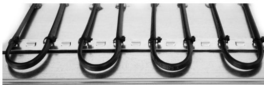
Монтажная лента, подклеенная специальной самоклеящейся лентой RT-L500-S-AL – длина рейки - 50 см
