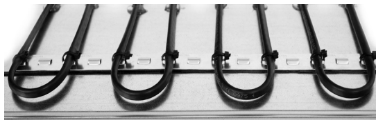
Listwa montażowa podklejona specjalną taśmą samoprzylepną RT-L500-S-AL – długość listwy – 50cm
